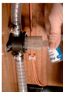
Grobschmutzfilter
